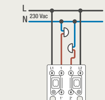
170-75015 / 170-75001 DUBBELE DRUKKNOP 2 x NORMAAL OPEN
