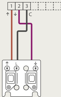
170-95915 / 170-95901 DUBBELE DRUKKNOP VOOR ELEKTRONISCHE STURINGEN (niet elektrisch gescheiden)
