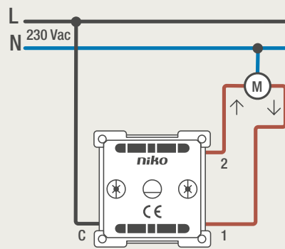
170-55901 / 170-35901 DRAAISCHAKELAAR 1 - 0 - 2 VOOR ROLLUIKEN IMPULSGEVEVER MET DRAAIBEDIENING (niet voor parallelwerking)
