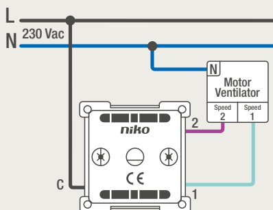
170-95915 / 170-95901 DUBBELE DRUKKNOP VOOR ELEKTRONISCHE STURINGEN (niet elektrisch gescheiden)
