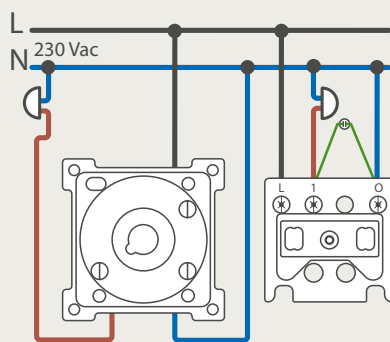
170-74001 170-70015 170-70001 DRUKKNOP VERLICHT (steeds drie geleiders)
