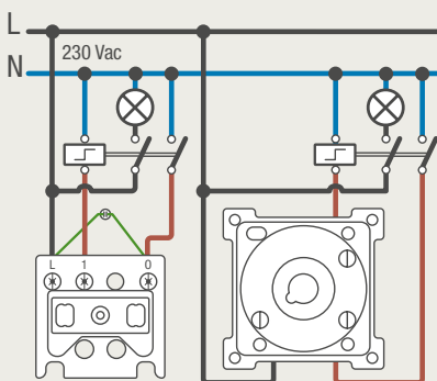
170-70015 170-70001 DRUKKNOP NORMAAL OPEN CONTROLE
