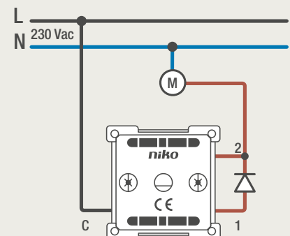
170-45901 DRAAISCHAKELAAR VOOR VENTILATOREN - 0, 1 EN 2
