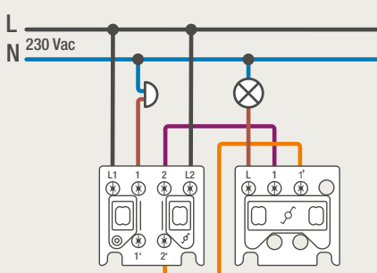
170-75615 170-71615 170-75601 170-71601 1 x WISSEL + 1 x NORMAAL OPEN
