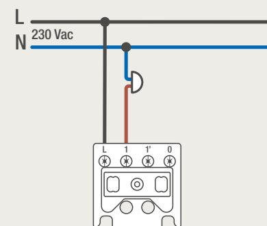
170-73015 / 170-73001 DRUKKNOP NORMAAL OPEN OF NORMAAL GESLOTEN
